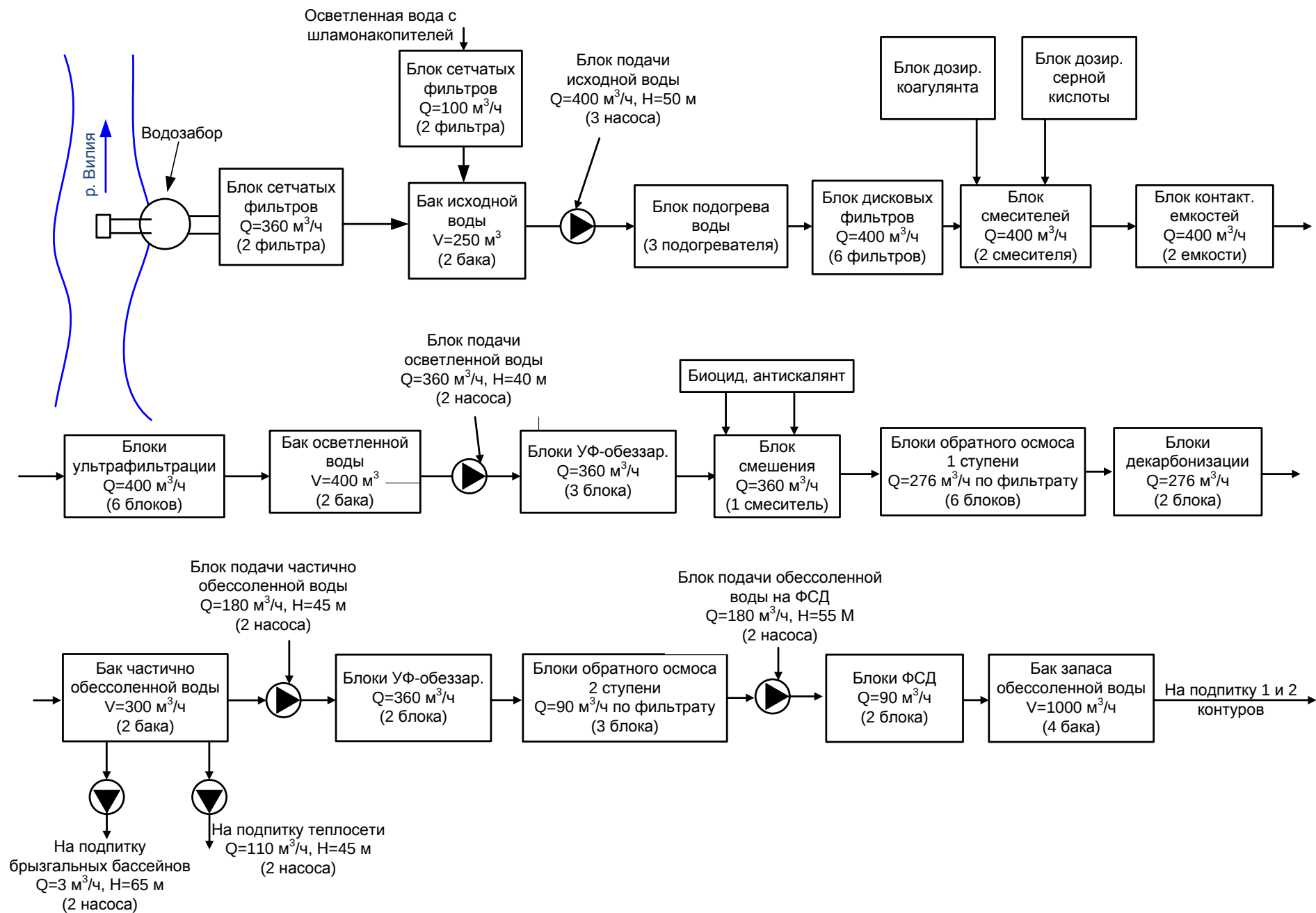
Рисунок 1. Принципиальная схема водоподготовительной установки на Белорусской АЭС ( Q – производительность, V – объем, H – напор)
